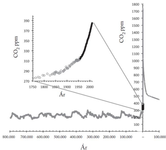
Mynd 13-1 Styrkur koltvíoxíðs í andrúmslofti 800.000 ár aftur í tíma og 100.000 ár fram á við. Styrkur koltvíoxíðs í andrúmslofti frá iðnbyltingu til ársins 2010 er dreginn út á innfelledu myndinni (Archer 2005; Keeling o.fl. 2012; MacFarling Meure o.fl. 2006; Lüthi o.fl. 2008).
