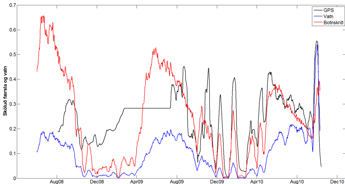
Mynd 1. Mæld færsla (GPS (m/d); svört lína), vatn (mm/klst; blá lína) og reiknað botnskrið (rauð lína) fyrir Breiðamerkurjökul.
