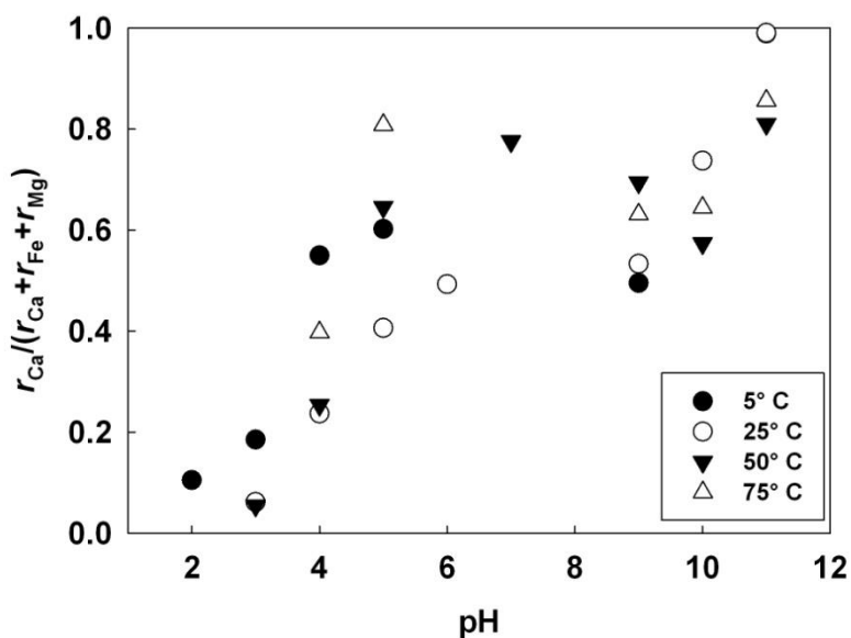
Mynd 1. Leysnihraði Ca sem hlutfall af leysnihraða tvígilda katjóna úr leysnitilraunum á kristölluðu basalti. Hlutfallslegur leysnihraði Ca eykst með hækkandi pH, sem gefur til kynna aukið vægi plagíóklas í leysni bersins.
