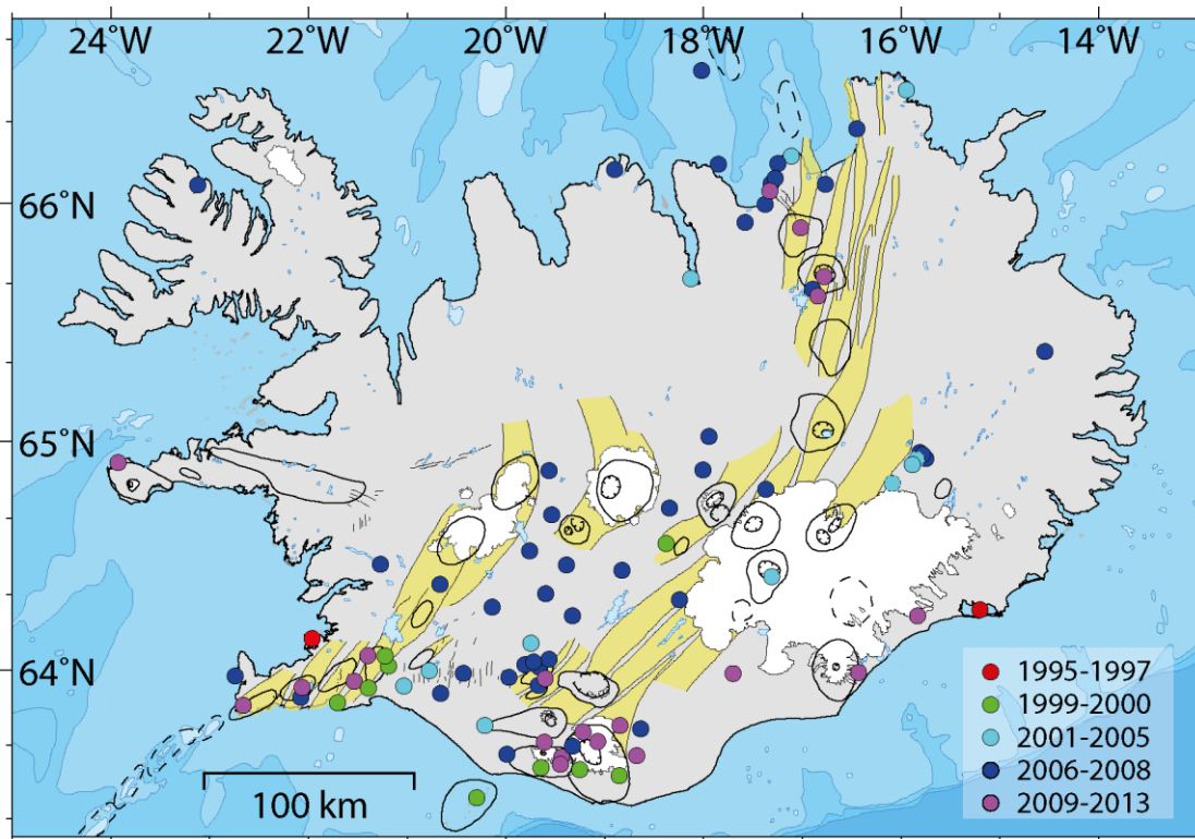
Mynd 1: Samfelldar GPS stöðvar á Ísland. Litur táknar hvenær stöðin hóf samfelldar mælingar.
